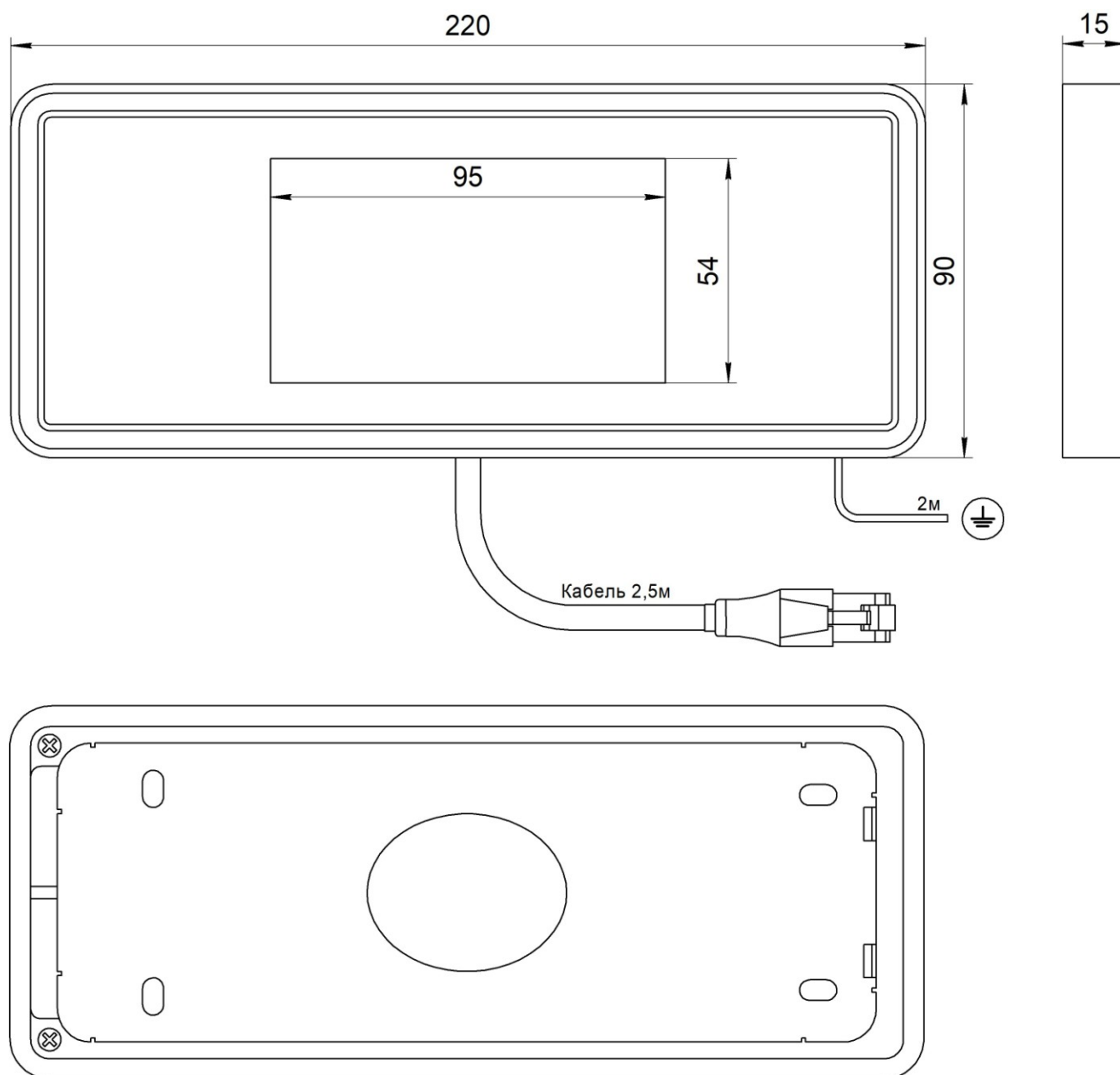
Рис.1 Внешний вид Табло накладное ОБСИДИАН (жгут RJ45) НШЕК.468232.139
